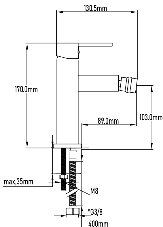
PLANO TÉCNICO
