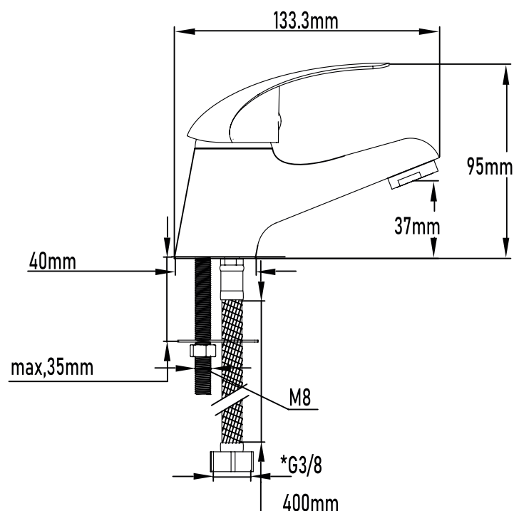
PLANO TÉCNICO
