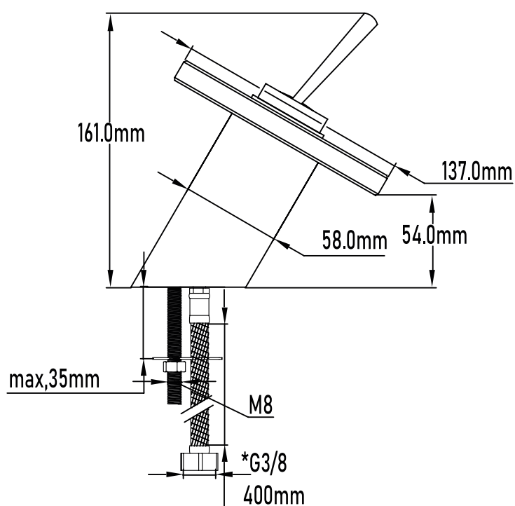
PLANO TÉCNICO
