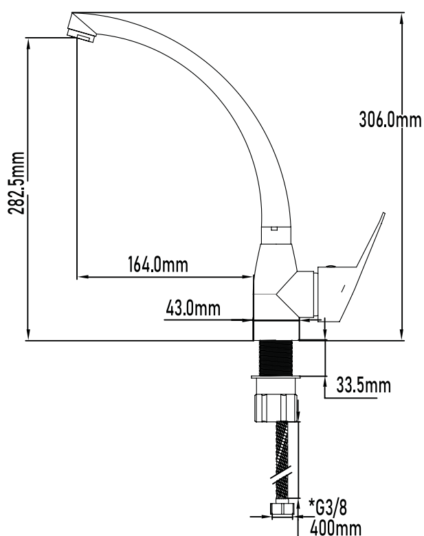
PLANO TÉCNICO
