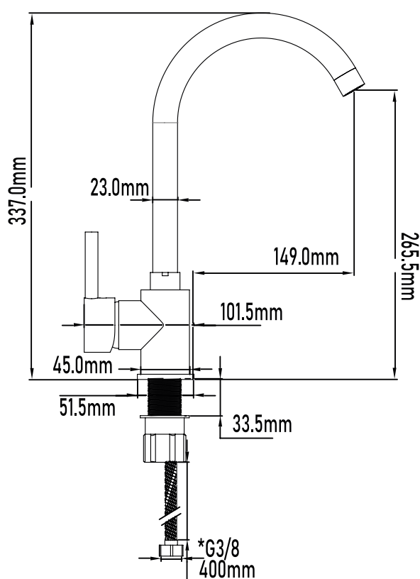
PLANO TÉCNICO
