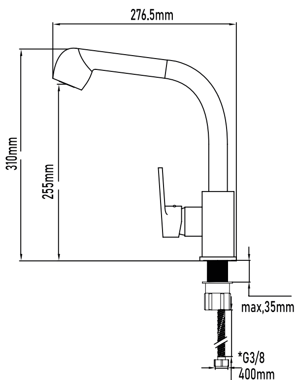
PLANO TÉCNICO
