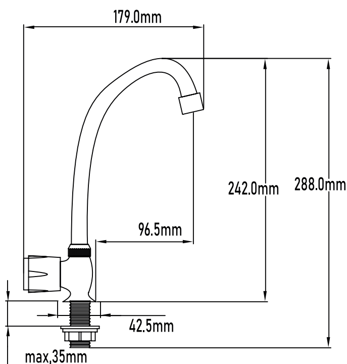
PLANO TÉCNICO
